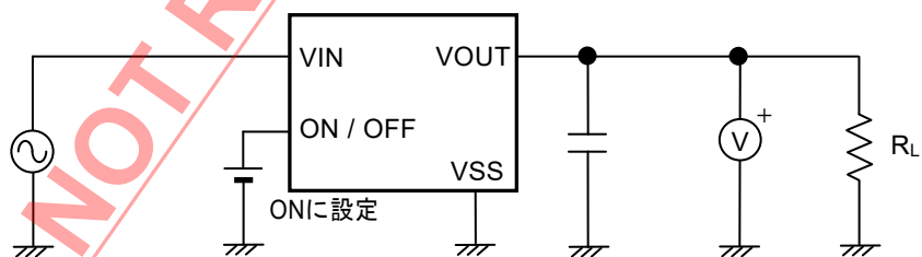
図13 測定回路5
