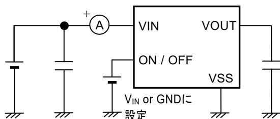
図10 測定回路2
