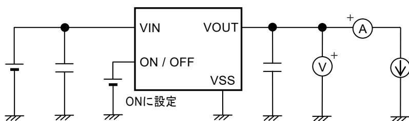
図9 測定回路1
