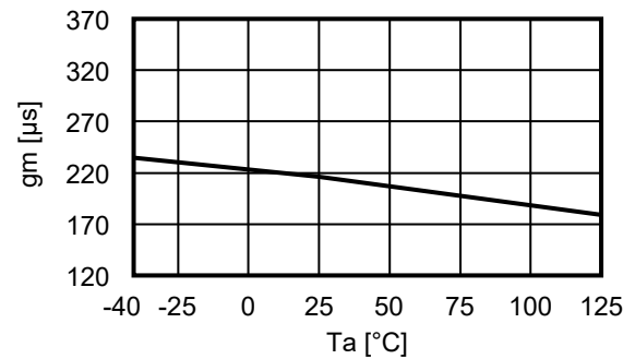
2.12 跨导误差放大电路 ( g_m ) – 温度 ( T_a )
