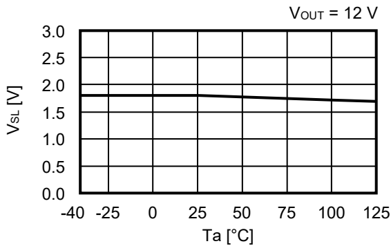
2.11 低电位输入电压 ( V_{SL} ) – 温度 ( T_a )
