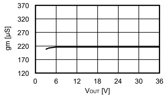
1.8 跨导误差放大电路 ( g_m ) – 输出电压 ( V_{OUT} )
