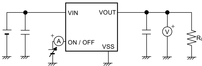
图11 测定电路4
