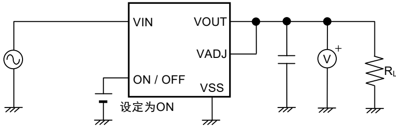
图18 测定电路11
