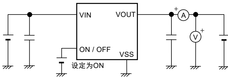
图10 测定电路3
