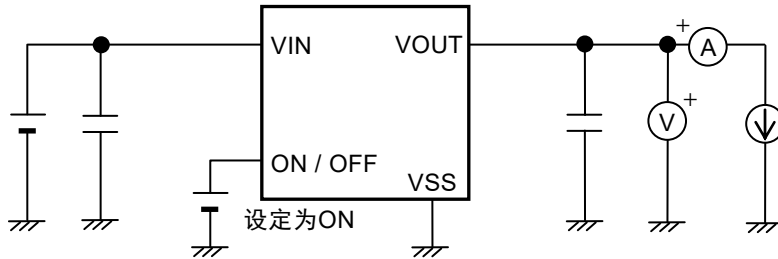
图8 测定电路1
