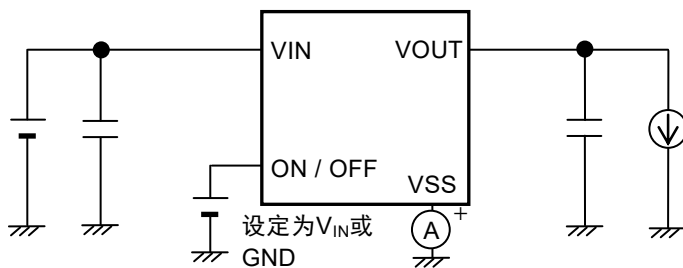
图9 测定电路2
