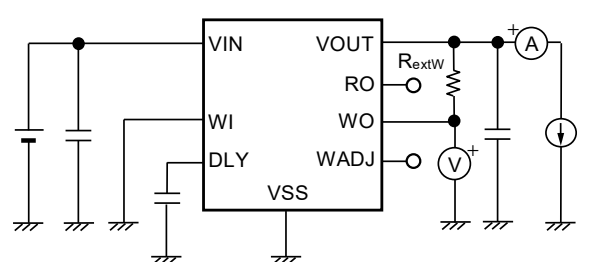
图27 测定电路6
