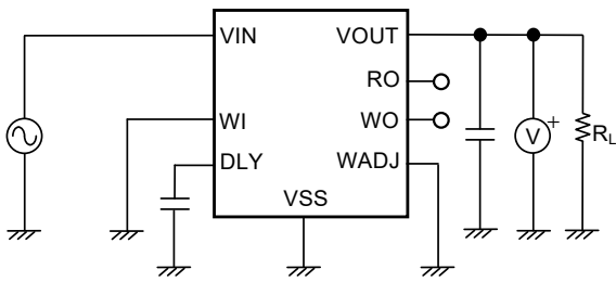
图24 测定电路3
