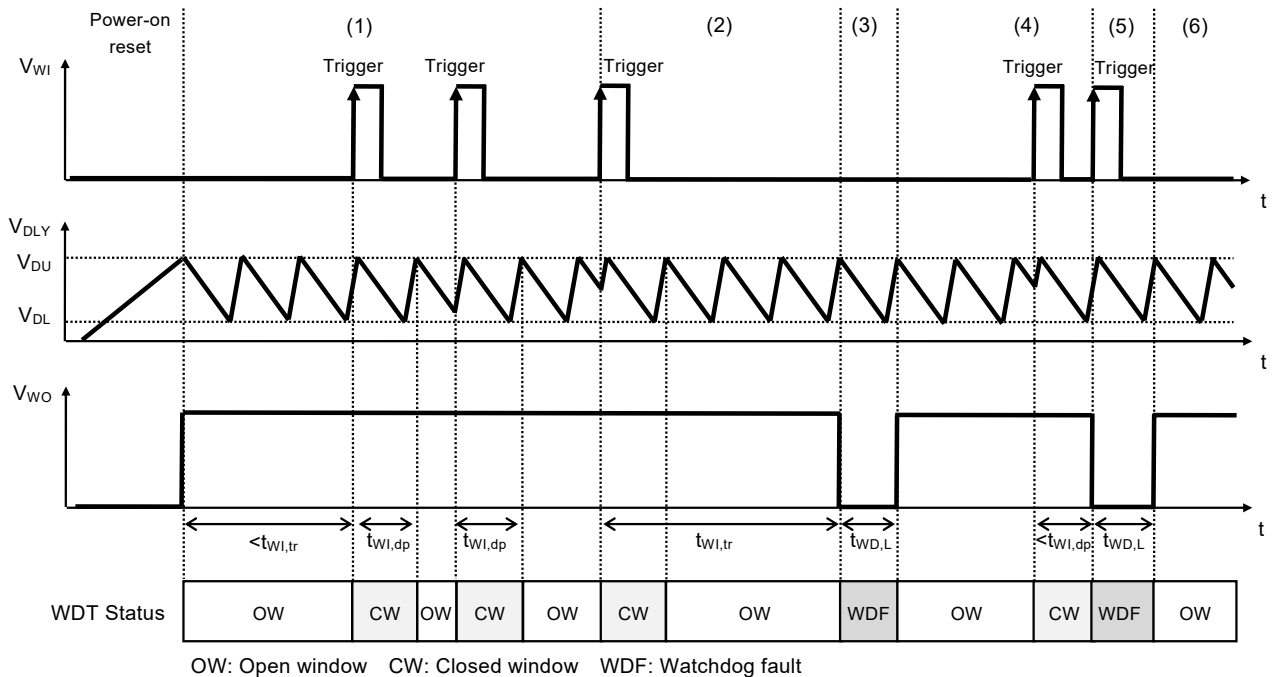
图37 看门狗定时器部分的时序图
