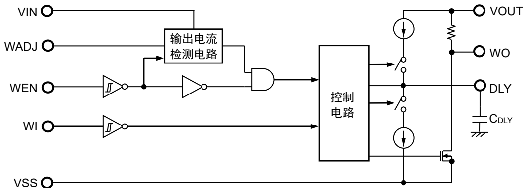
图39 看门狗定时器部分的工作说明图
