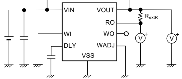
图25 测定电路4
