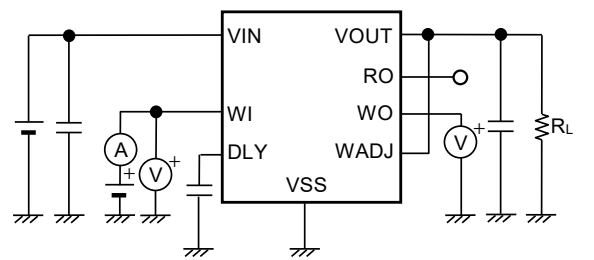
图29 测定电路8
