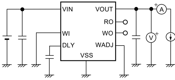
图22 测定电路1
