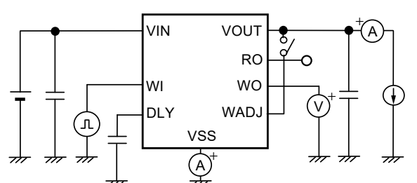
图31 测定电路10
