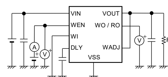
图20 测定电路9
