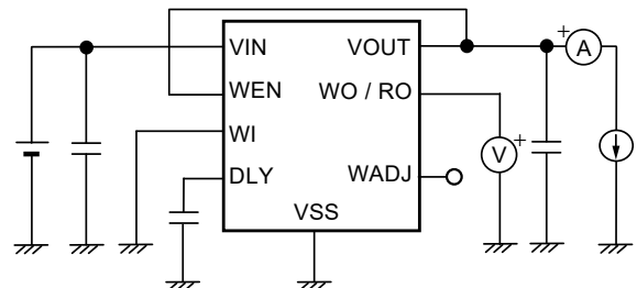
图17 测定电路6
