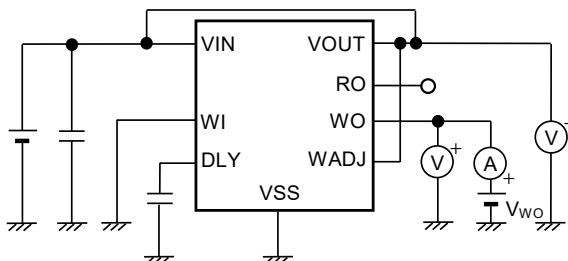
图30 测定电路9
