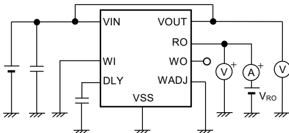
图26 测定电路5
