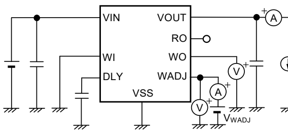
图28 测定电路7
