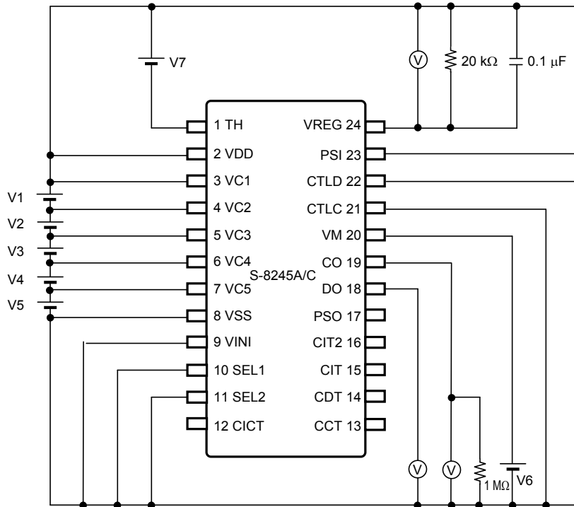
图4 测定电路2
