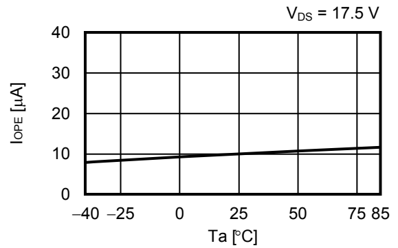
1.2 I_{OPE} - Ta
