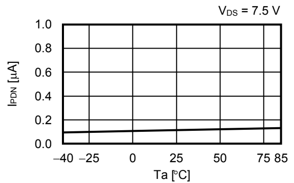
1.4 I_{PDN} - Ta
