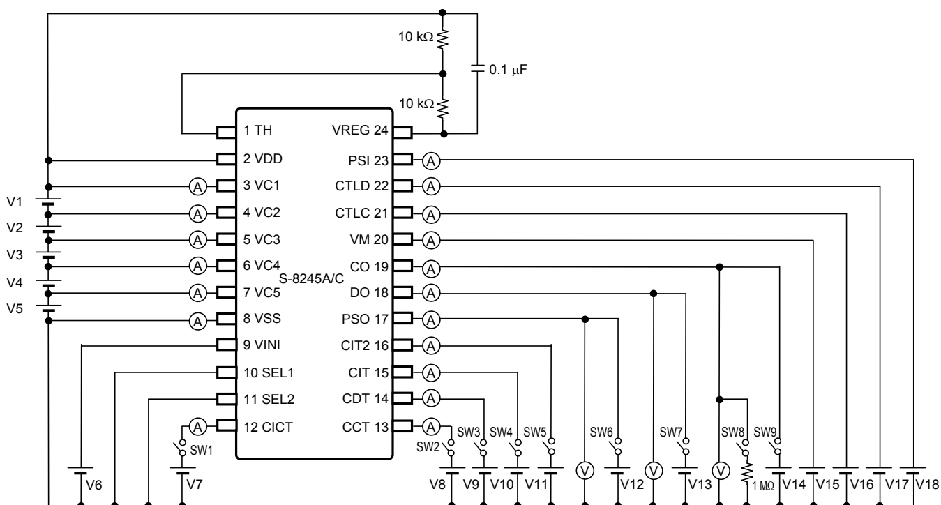
图3 测定电路1
