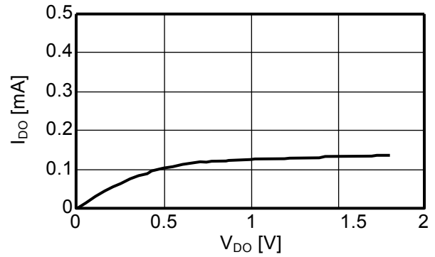
DO端子吸收电流特性 V_{DD} = 1.8\text{ V}, V_M = V_{SS} = 0\text{ V}
