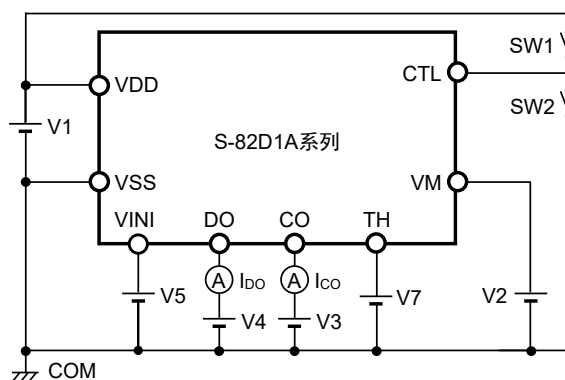
图6 测定电路4
