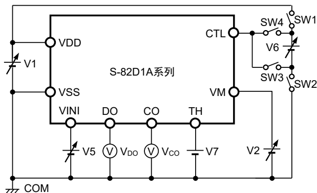
图4 测定电路2
