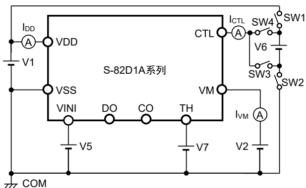
图5 测定电路3
