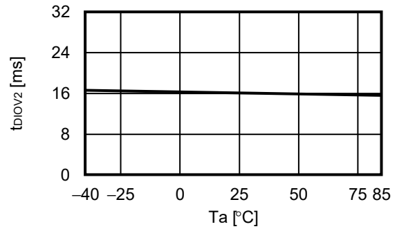
3.6 t_{DIOV2} - T_a
