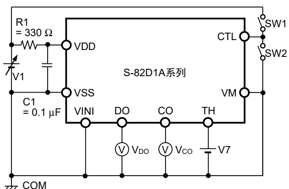
图3 测定电路1
