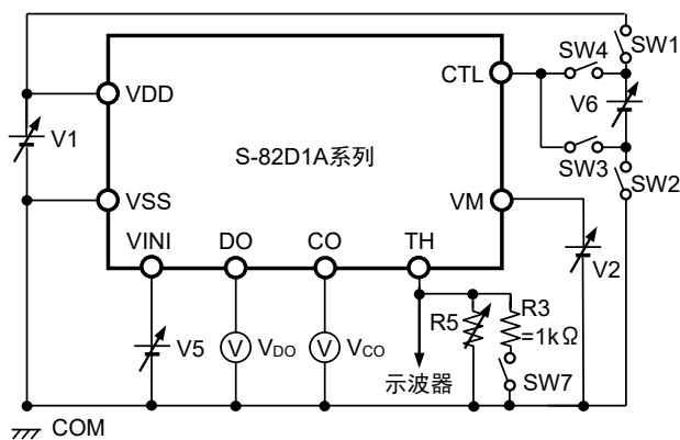
图6 测定电路4
