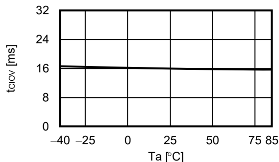
3.10 t_{CLOV} - T_a
