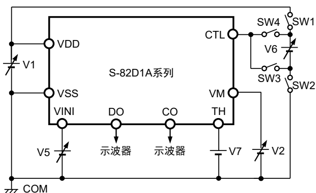
图7 测定电路5
