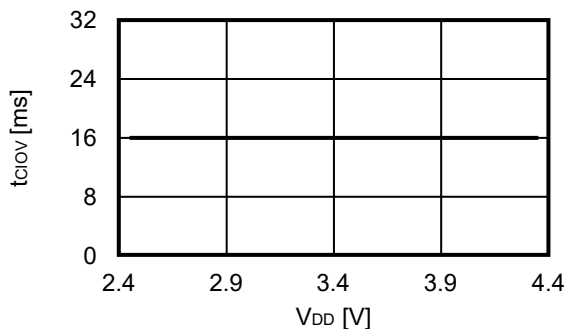
3.9 t_{CLOV} - V_{DD}
