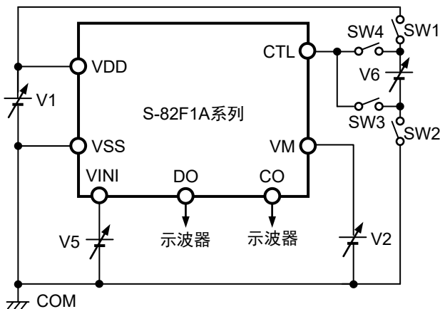
图7 测定电路5
