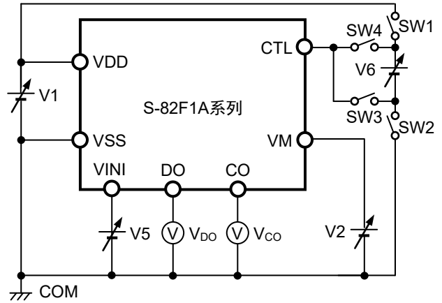
图4 测定电路2
