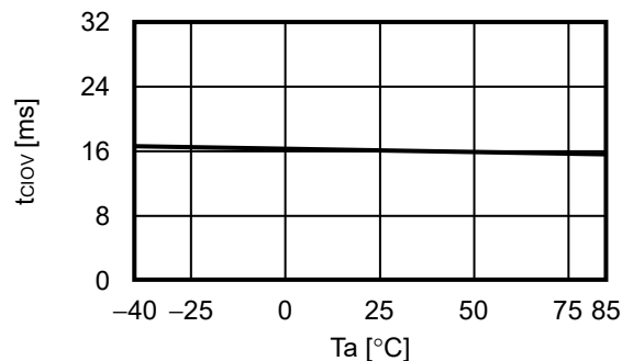
3.10 t_{CLOV} - T_a
