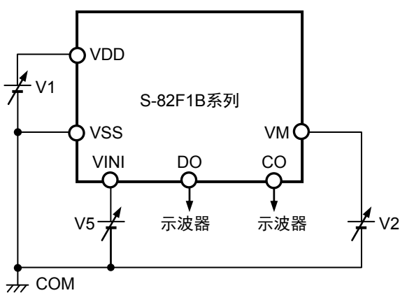
图7 测定电路5
