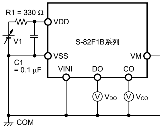
图3 测定电路1
