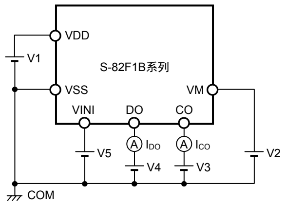
图6 测定电路4
