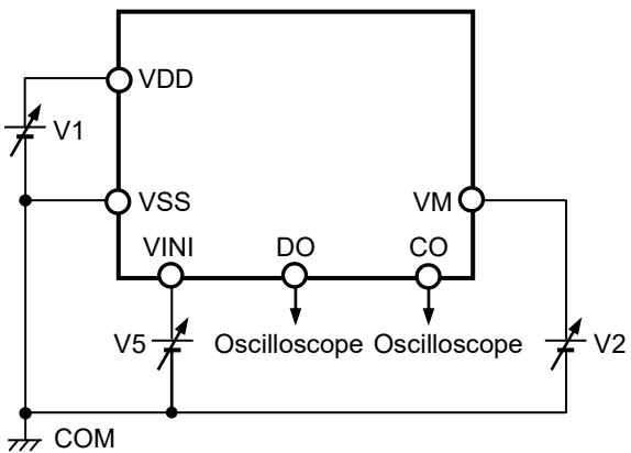
图8 测定电路5
