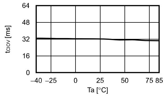
3.10 t_{CI0V} - T_a
