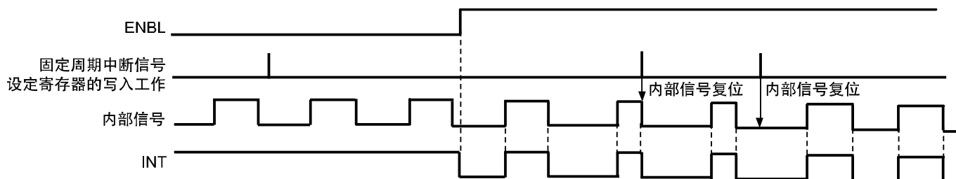
图12 INT端子的输出时序例2
