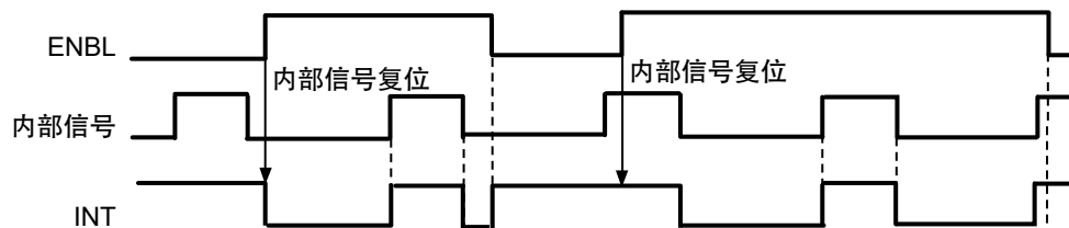
图11 INT端子的输出时序例1
