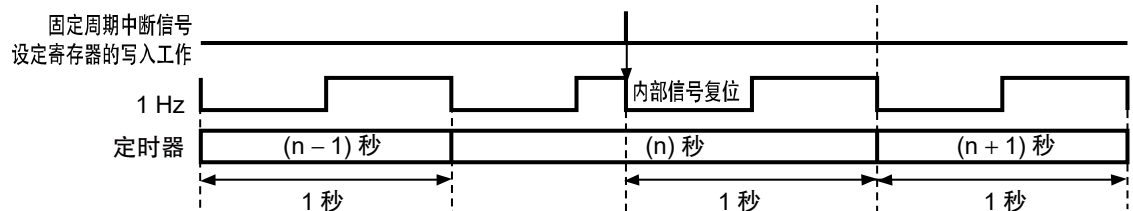
图13 定时器的递增计数和内部信号复位
