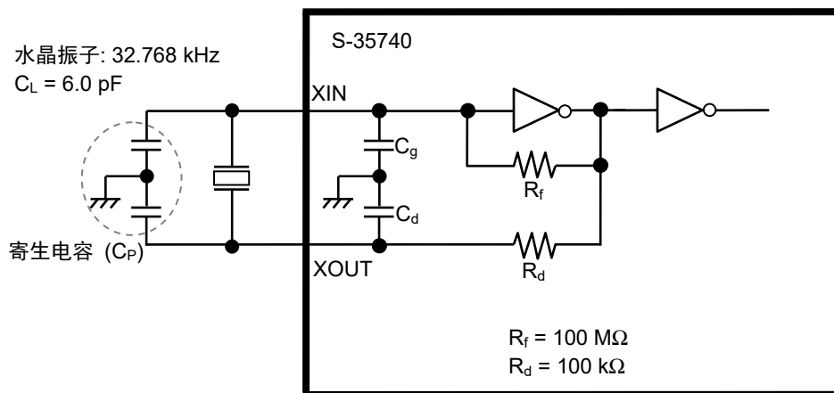
图27 晶振电路的构成
