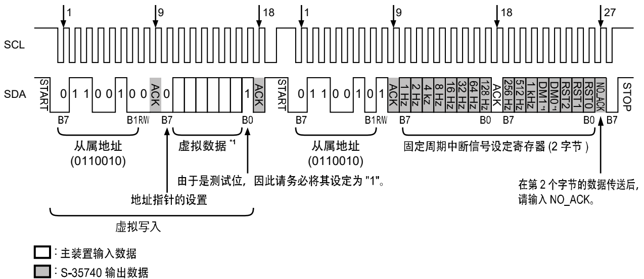
图21 固定周期中断信号设定寄存器的读出时序
