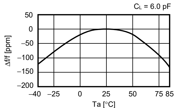
8. 振荡频率 – 温度特性
