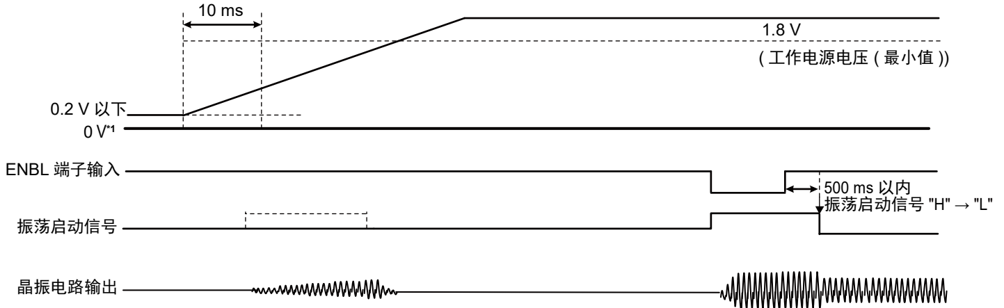
图25 ENBL端子 = "H" 时的电源电压上升
