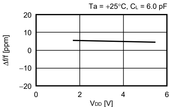
7. 振荡频率 – 电源电压特性
