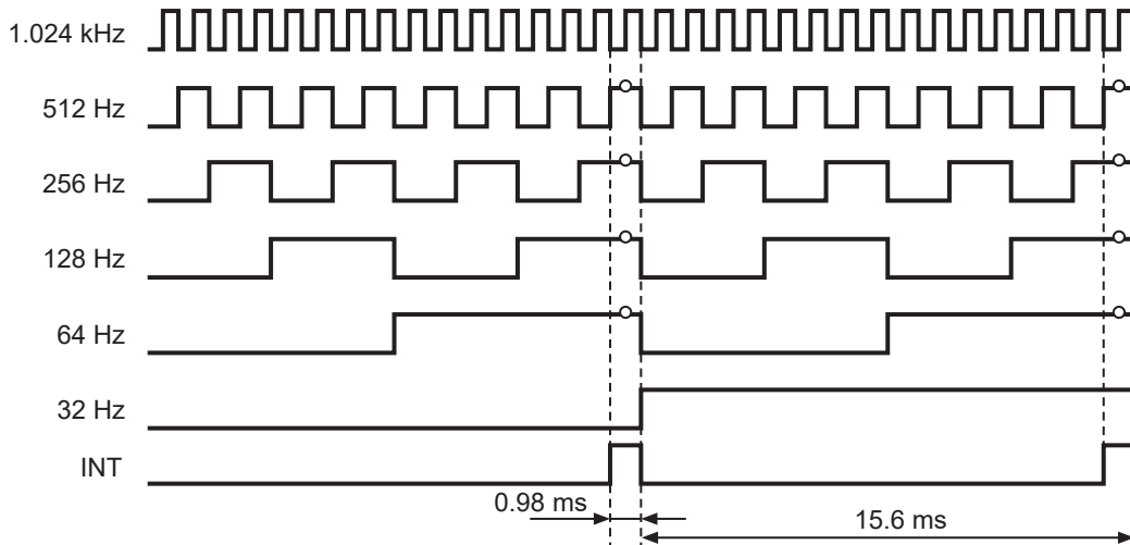
图10 固定周期中断信号输出例
