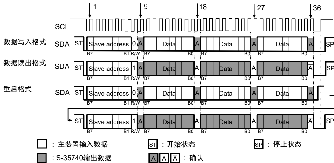
图18 串行接口的数据传送格式
