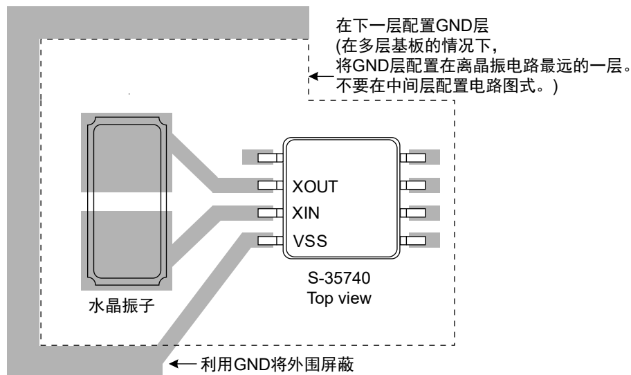
图28 连接布局图的推荐例
