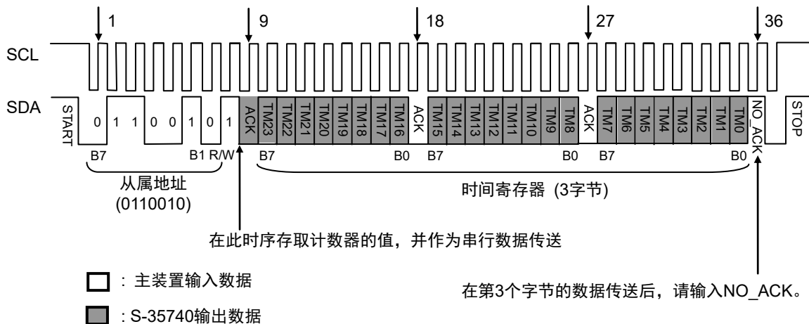
图19 时间寄存器的读出时序
