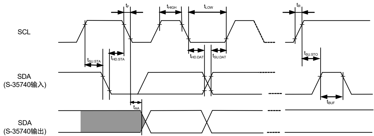
图8 总线时序
