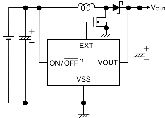
图 19 使用 MOS FET(N 沟道)型产品的电路示例
