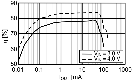
(d) 输出电流( I_{OUT} )—效率( \eta )特性
