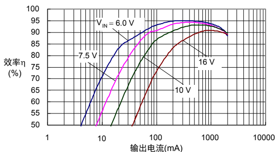
(7) S-8533A50AFT (CPH6302/CPH6402)
