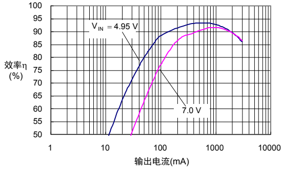
(25) S-8533A33AFT (CPH6303/CPH6403)
