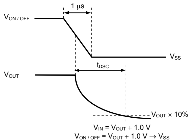
图25 放电时间的测定条件
