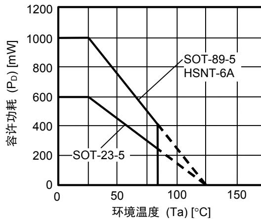
图12 封装容许功耗
