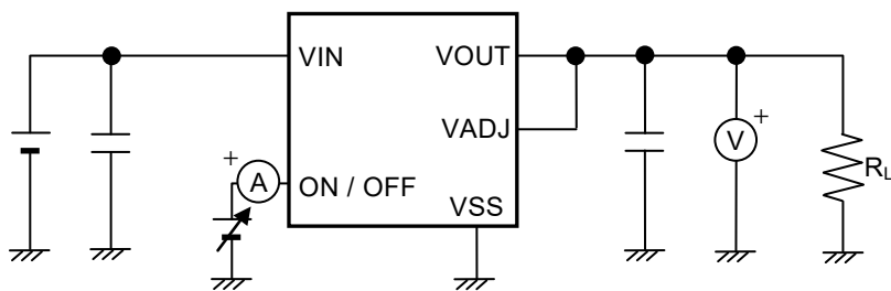
图14 测定电路10
