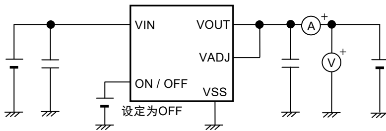
图16 测定电路12
