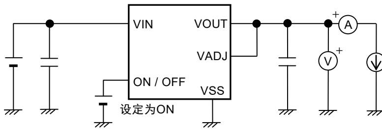
图11 测定电路7
