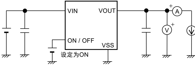
图5 测定电路1
