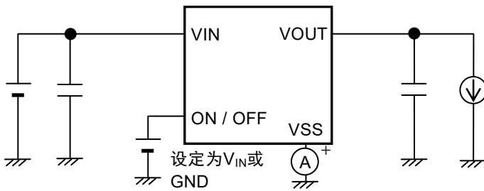
图6 测定电路2
