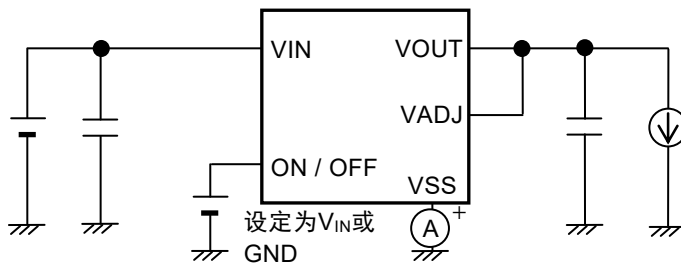
图12 测定电路8
