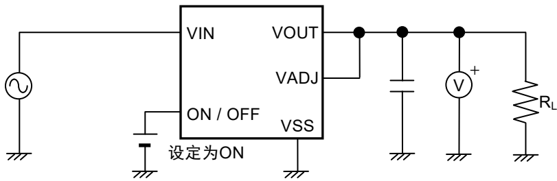
图15 测定电路11
