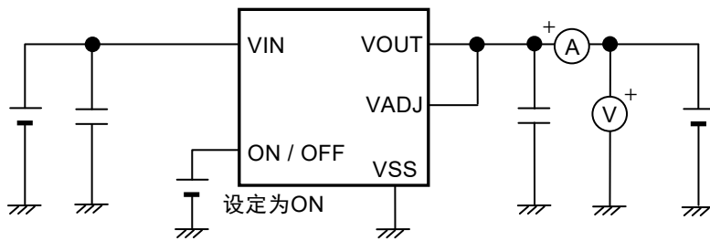
图13 测定电路9
