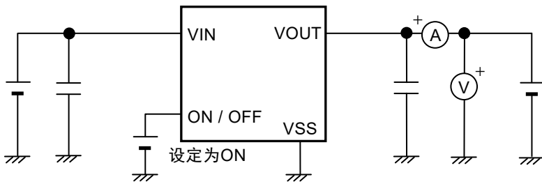
图7 测定电路3
