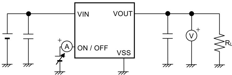
图8 测定电路4
