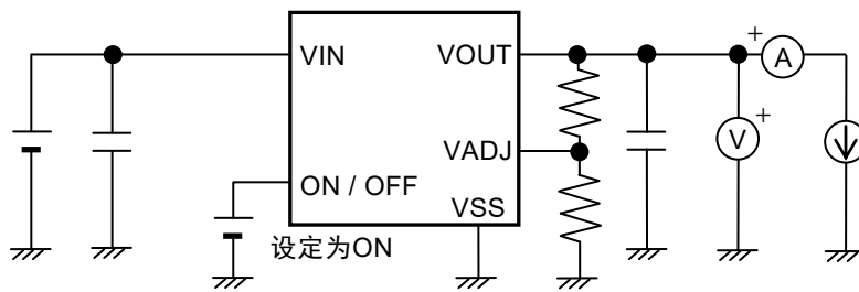
图17 测定电路13
