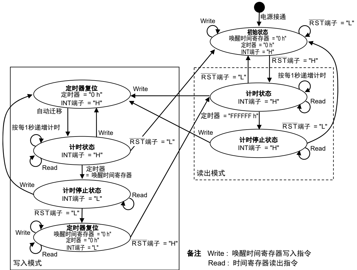
图16 握手协议终止的状态迁移图 (S-35710C011 / N沟道开路漏极输出)
