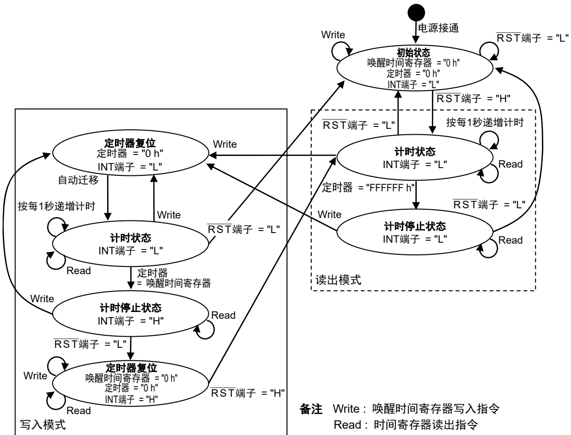
图17 握手协议终止的状态迁移图 (S-35710B011 / CMOS输出)
