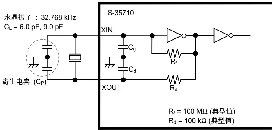
图33 晶振电路构成
