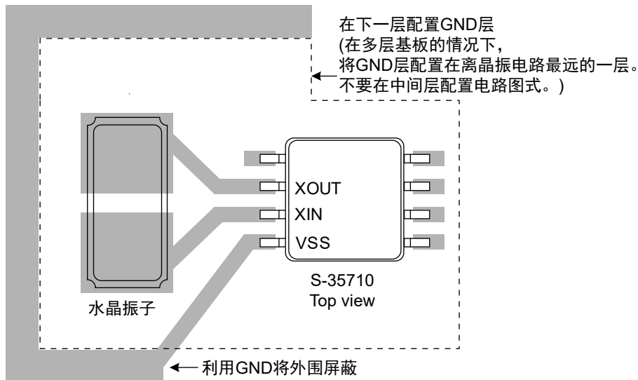
图34 连接布局图的推荐例
