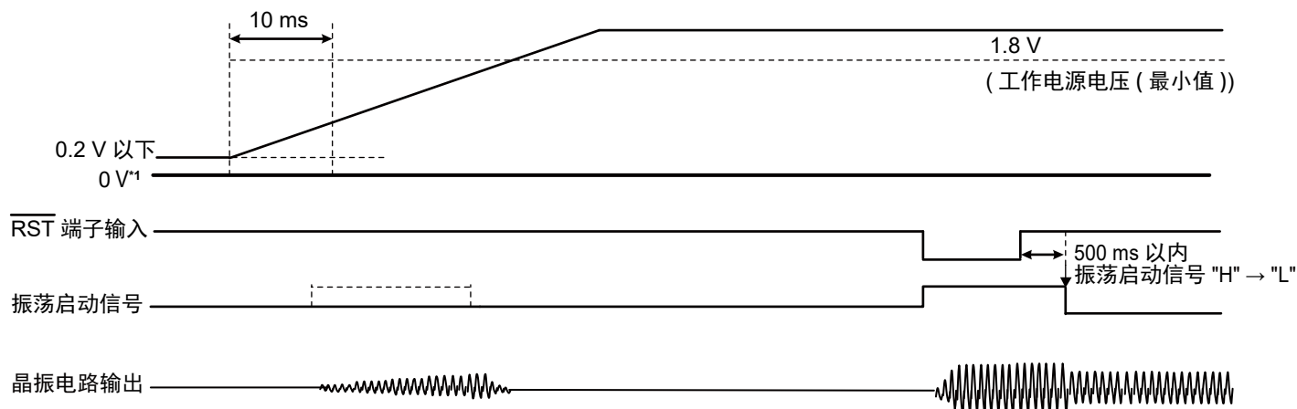
图29 \overline{\text{RST}} 端子 = "H" 时的电源电压上升
