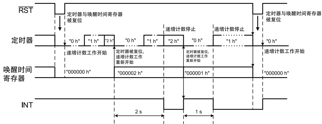
图12 握手协议终止的输出时序例 (S-35710C011 / N沟道开路漏极输出)
