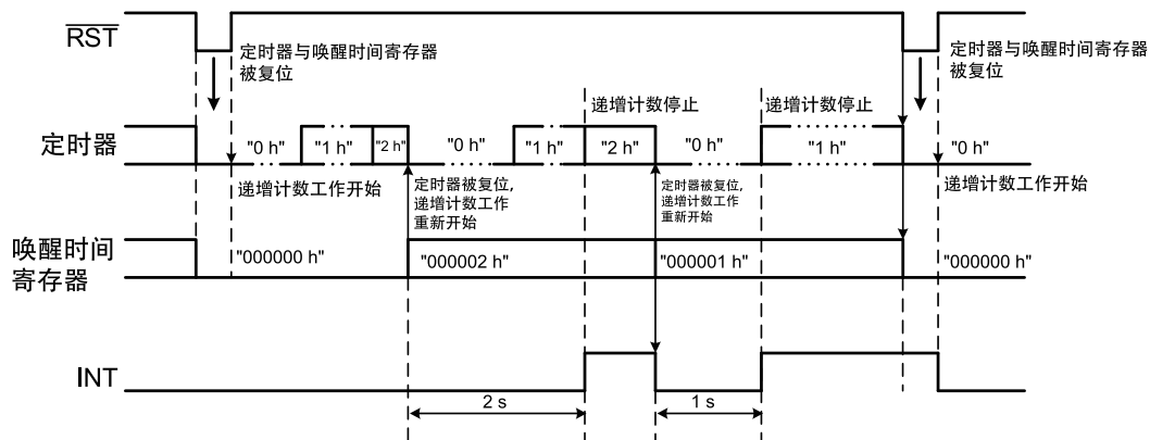
图13 握手协议终止的输出时序例 (S-35710B011 / CMOS输出)
