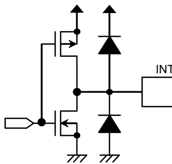
图8 INT端子 (S-35710B011 / CMOS输出)
