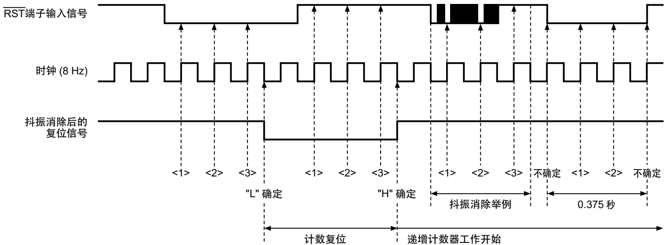
图30 抖振消除的时序图例
