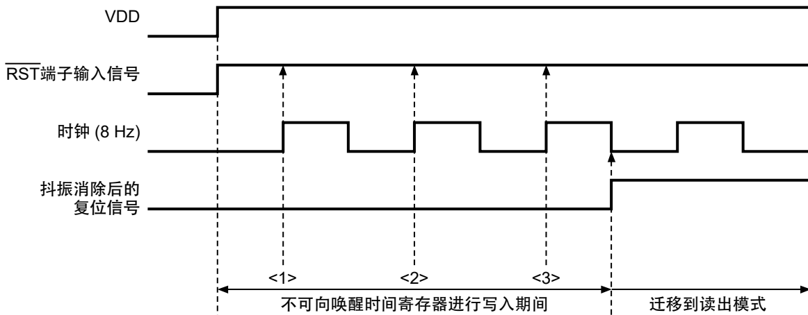
图31 电源接通时的时序图
