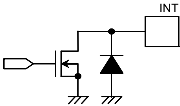
图7 INT端子 (S-35710C011 / N沟道开路漏极输出)
