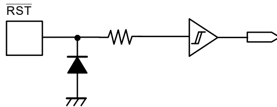
图6 \overline{\text{RST}} 端子 (S-35710C011 / 无上拉电阻)
