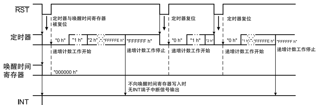
图14 不向唤醒时间寄存器写入时 (S-35710C011 / N沟道开路漏极输出)
