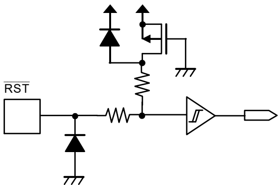
图5 \overline{\text{RST}} 端子 (S-35710B011 / 有上拉电阻)
