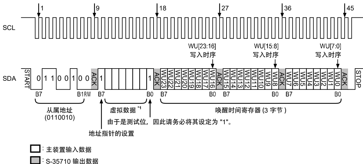
图24 唤醒时间寄存器的写入时序
