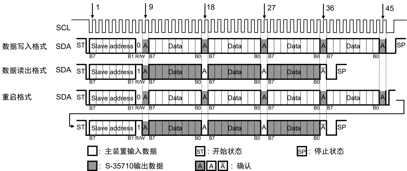
图22 串行接口的数据传送格式
