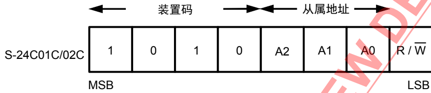
图13 装置地址
