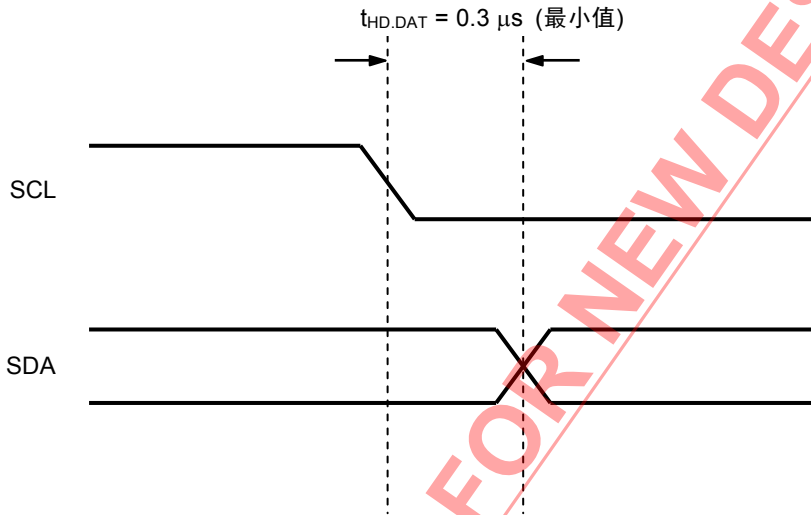
图30 S-24C01C/02C的数据保持时间
