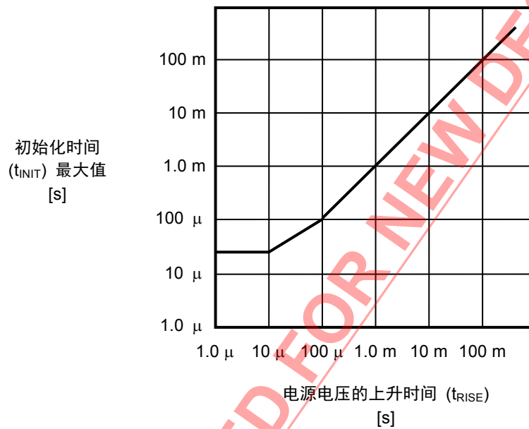
图29 S-24C01C/02C的初始化时间
