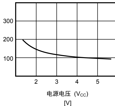
图31 SDA端子和SCL端子的噪声抑制时间
