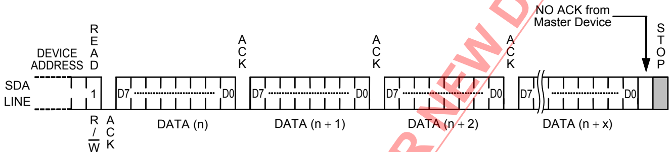
图20 顺序读出
