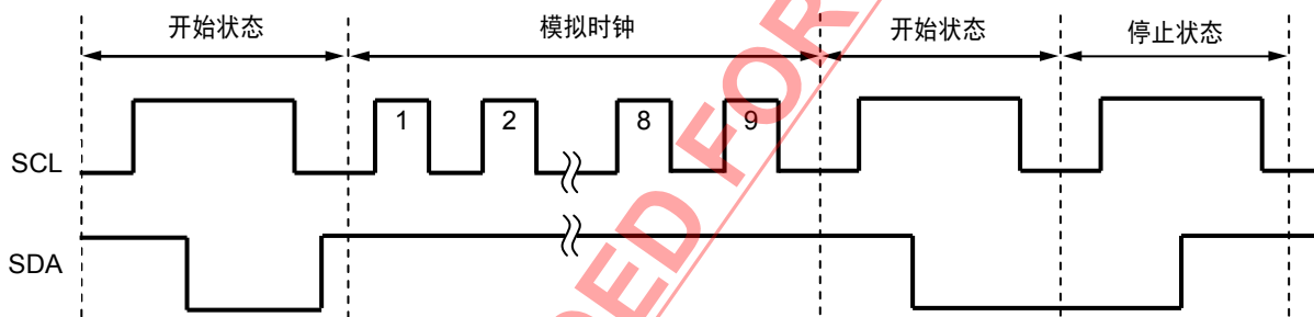
图26 S-24C01C/02C的复位方法
