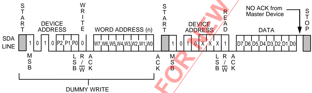
图19 随机读出
