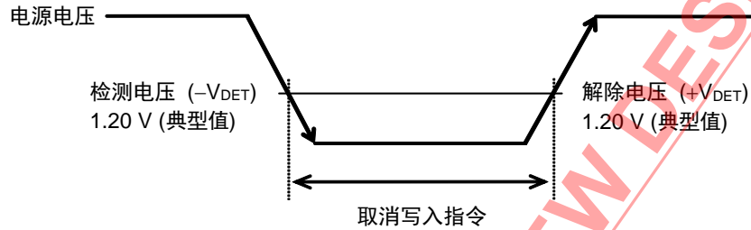
图21 低电源电压时的工作
