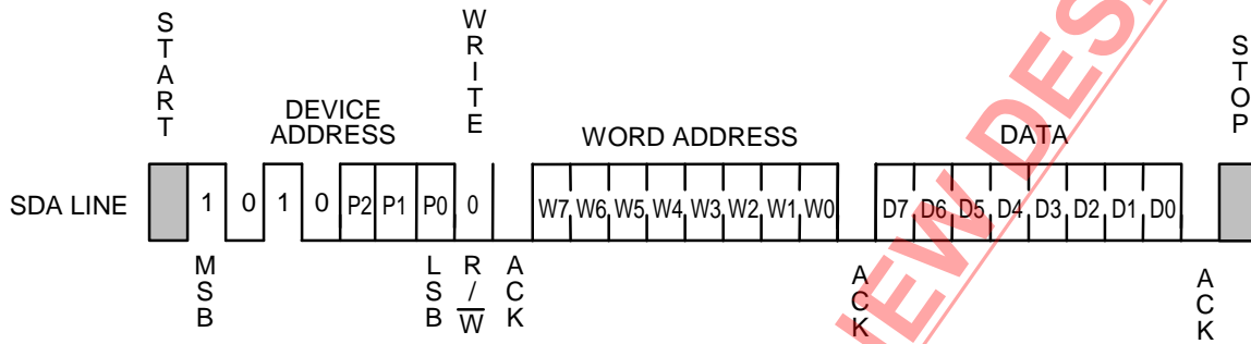
图14 字节写入
