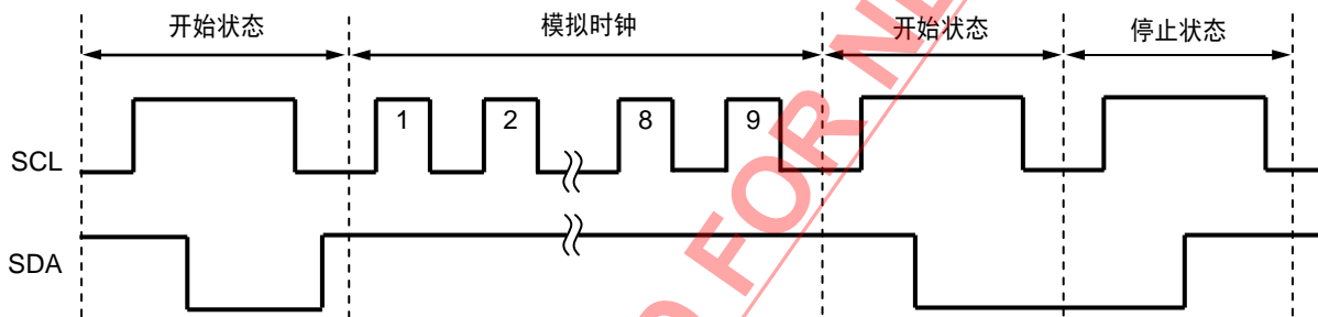
图25 S-24C16C的复位方法
