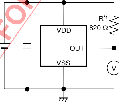
图8 测定电路4
