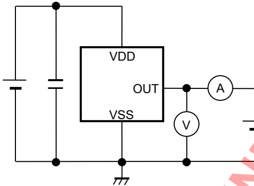
图7 测定电路3
