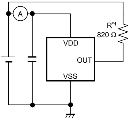
图5 测定电路1
