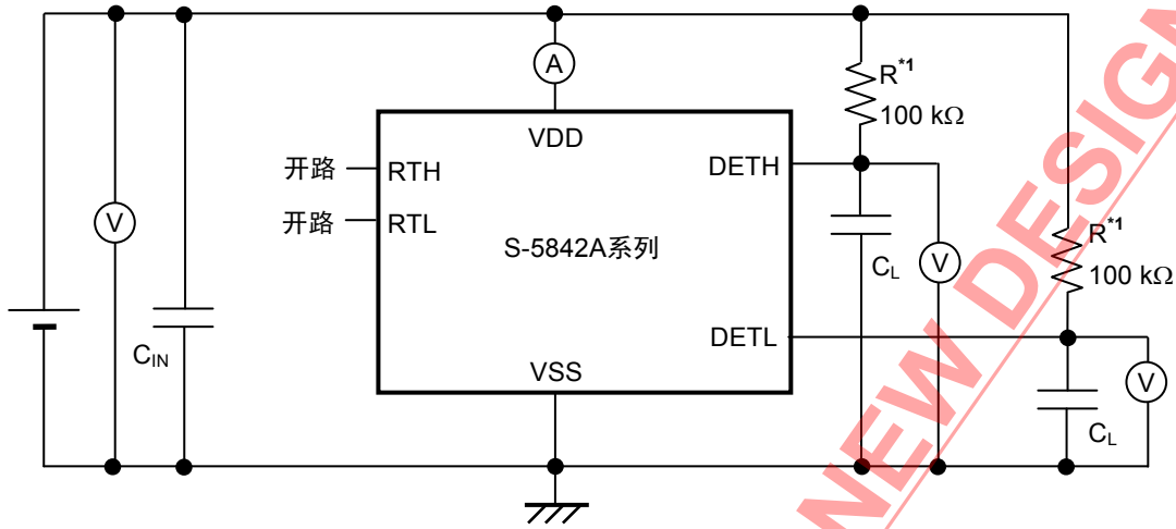
图7 测定电路1
