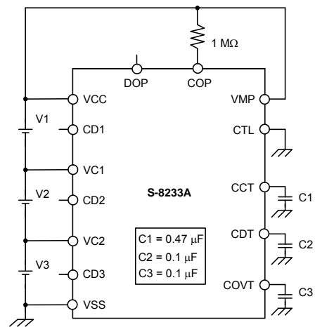
测定电路6
