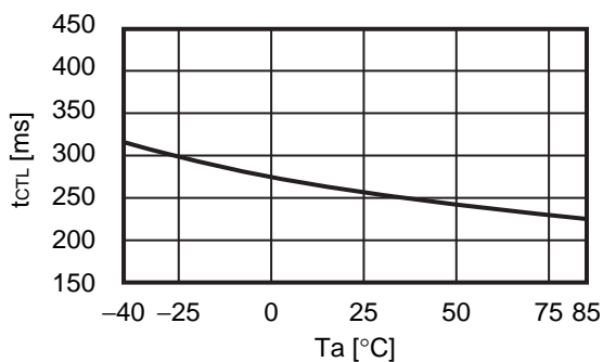
3.9 t_{CTL} - T_a
