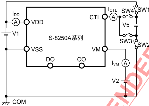
图6 测定电路3
