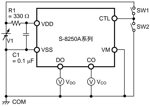
图4 测定电路1
