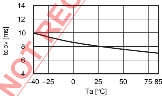
3.7 t_{CIOV} - T_a
