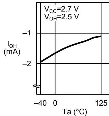
1.24 高电位输出电流 I_{OH} 一周围温度 T_a
