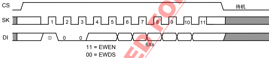
图17 允许或禁止写入定时 (S-93A56A, S-93A66A)
