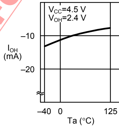
1.22 高电位输出电流 I_{OH} 一周围温度 T_a
