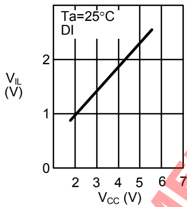
1.33 低电位输入电压 V_{IL} —电源电压 V_{CC}
