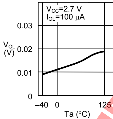
1.21 低电位输出电压 V_{OL} 一周围温度 T_a
