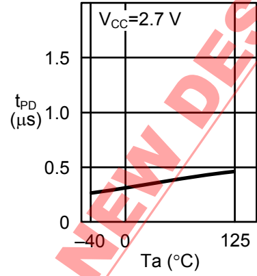
2.8 数据输出延迟时间 t_{PD} —周围温度 T_a
