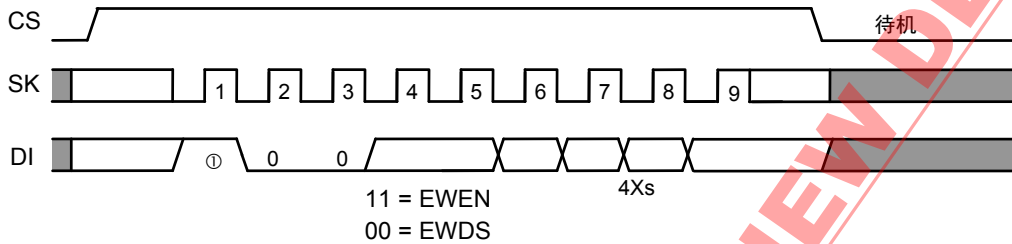
图16 允许或禁止写入定时 (S-93A46A)
