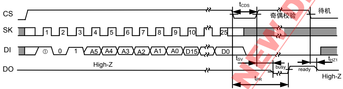
图8 数据写入定时 (S-93A46A)
