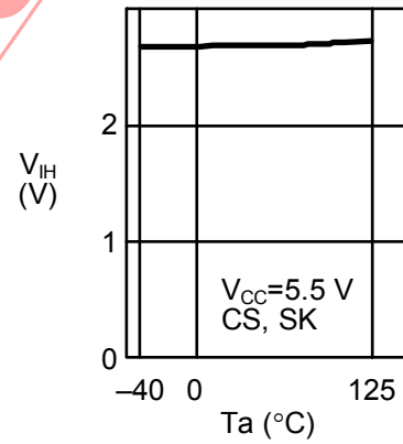
1. 28 高电位输入电压 V_{IH} —周围温度 T_a
