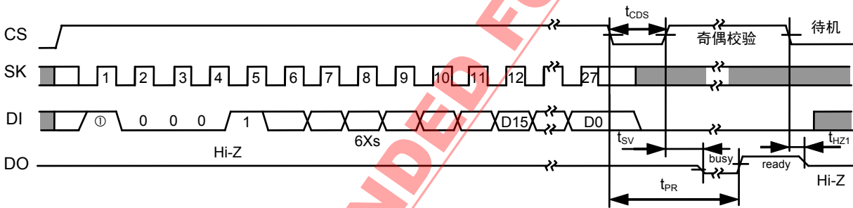
图13 全部写入定时 (S-93A56A, S-93A66A)
