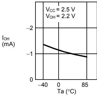
1.25 高电位输出电流 I_{OH} —周围温度 T_a
