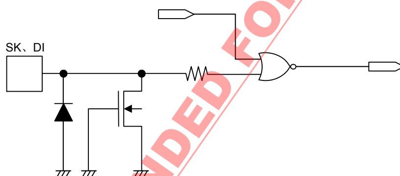
图15 SK、DI端子
