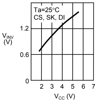
1.27 输入反转电压 V_{INV} —电源电压 V_{CC}
