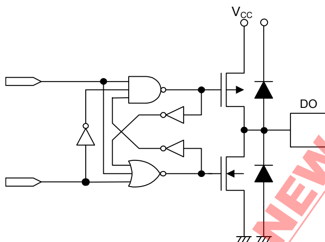
图26 DO端子
