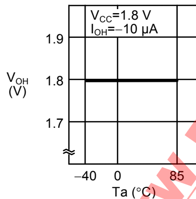
1. 20 高电位输出电压 V_{OH} —环境温度 T_a
