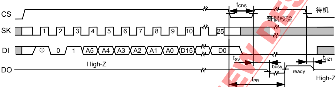
图10 数据写入定时 (S-93L46A)
