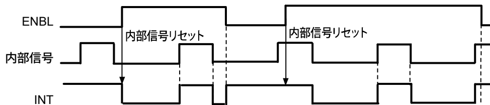
図14 INT端子の出力タイミング例1 (CMOS出力)
