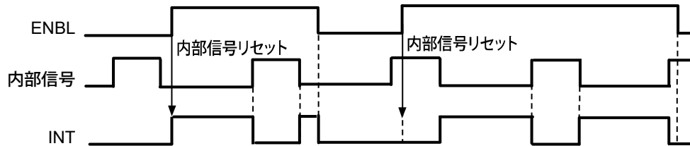
図13 INT端子の出力タイミング例1 (Nchオープンドレイン出力)
