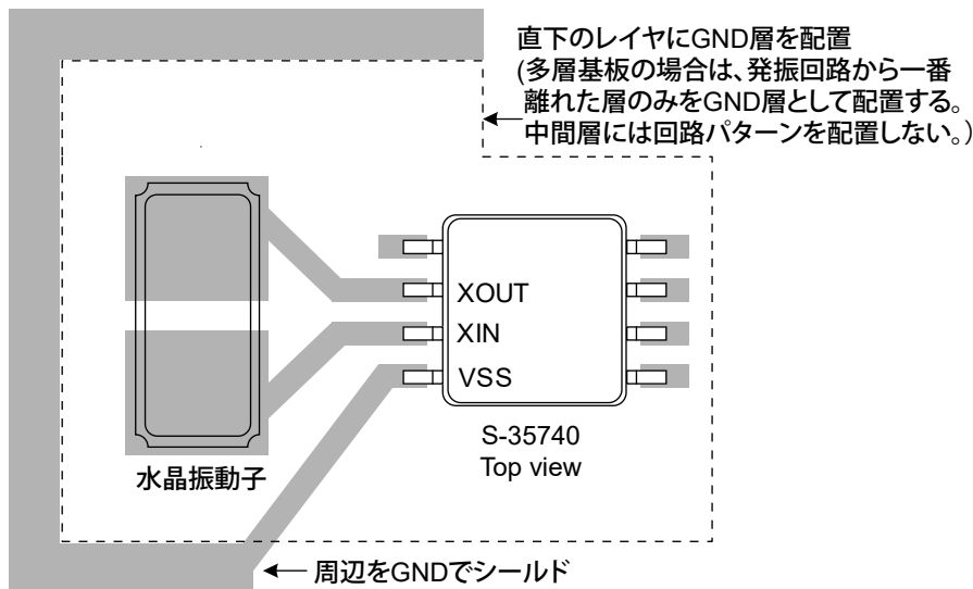
図32 接続パターン図の推奨例
