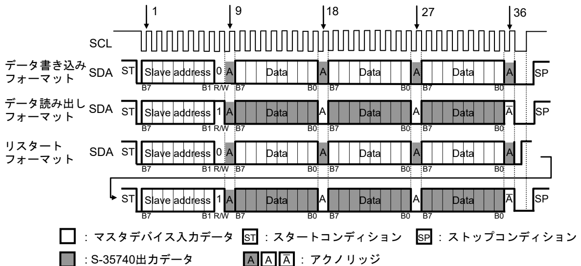
図22 シリアルインタフェースのデータ転送フォーマット
