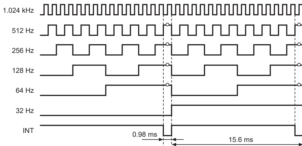
図11 定周期割り込み信号出力の例 (Nchオープンドレイン出力)
