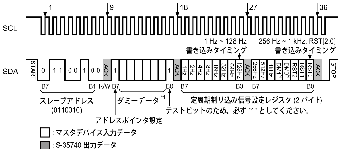
図24 定周期割り込み信号設定の書き込みタイミング
