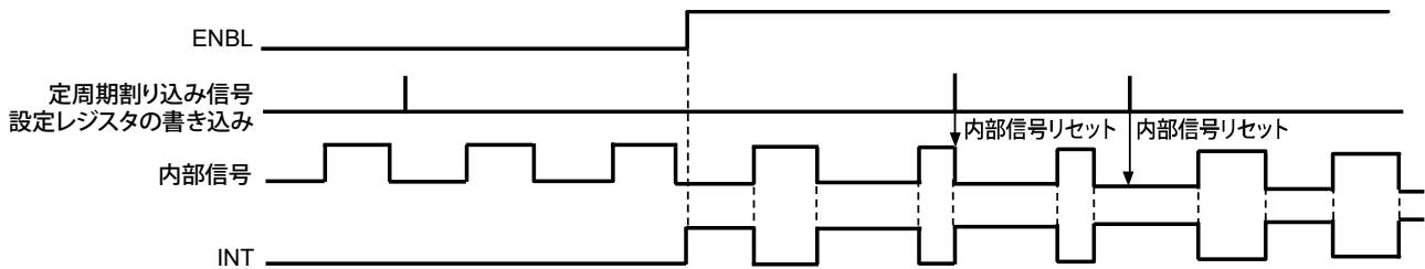
図15 INT端子の出力タイミング例2 (Nchオープンドレイン出力)
