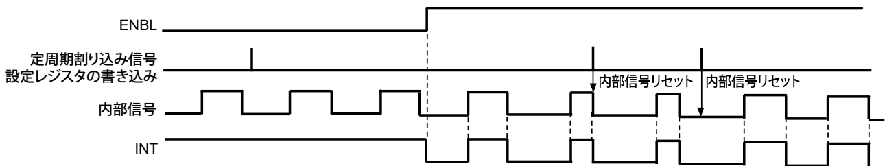
図16 INT端子の出力タイミング例2 (CMOS出力)
