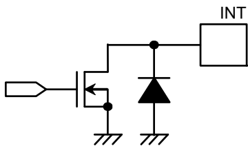
図6 INT端子 (Nchオープンドレイン出力)
