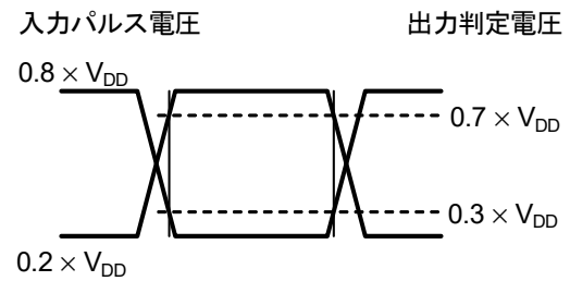
図8 AC測定入出力波形
