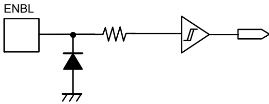
図5 ENBL端子
