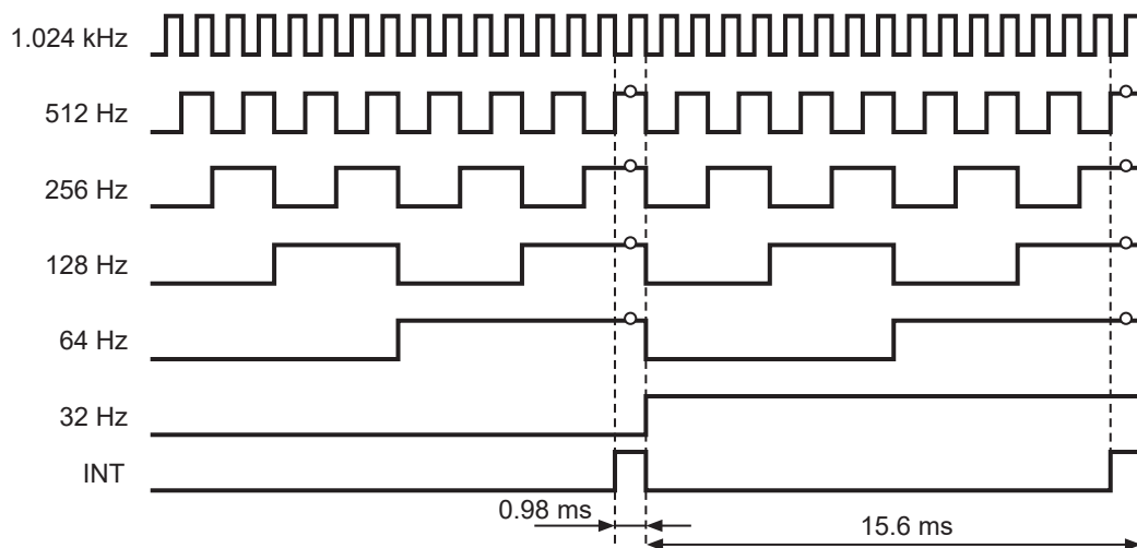
図12 定周期割り込み信号出力の例 (CMOS出力)
