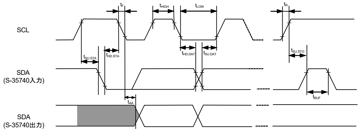
図9 バスタイミング
