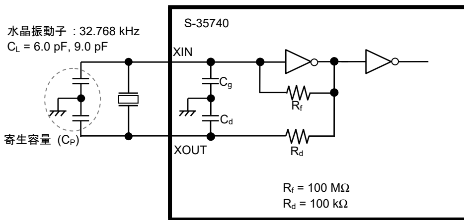
図31 水晶発振回路の構成
