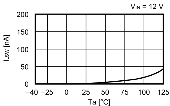
2.13 ロウサイドパワー-MOS FETリーク電流 ( I_{LSW} ) – 温度 ( T_a )
