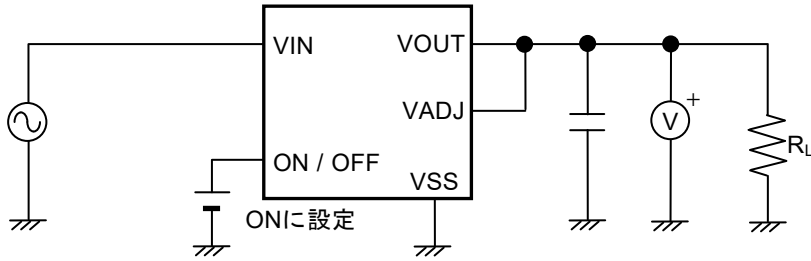
図18 測定回路11
