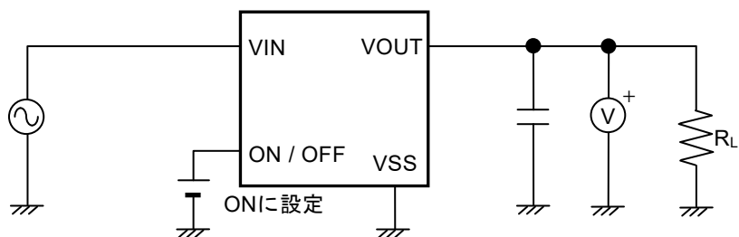
図12 測定回路5
