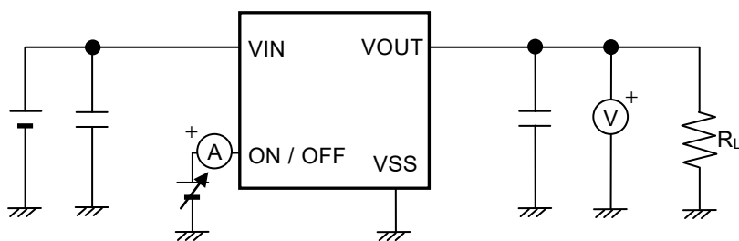
図11 測定回路4
