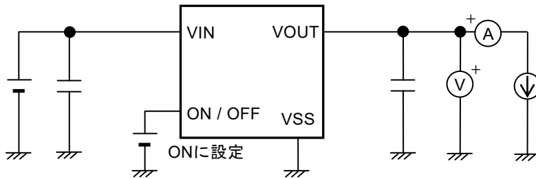
図8 測定回路1
