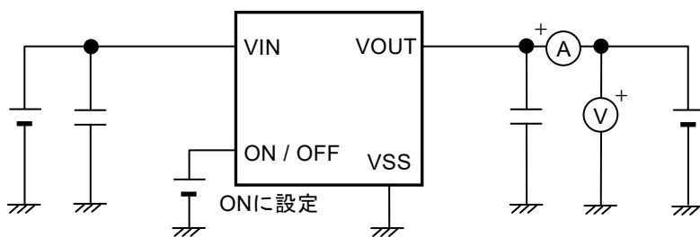
図10 測定回路3
