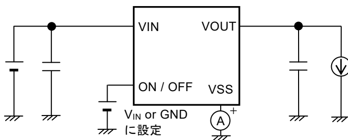
図9 測定回路2
