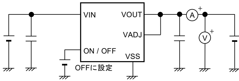
図19 測定回路12
