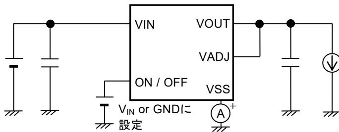
図15 測定回路8
