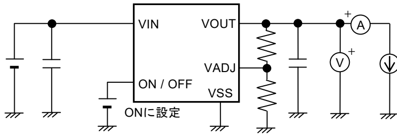
図20 測定回路13
