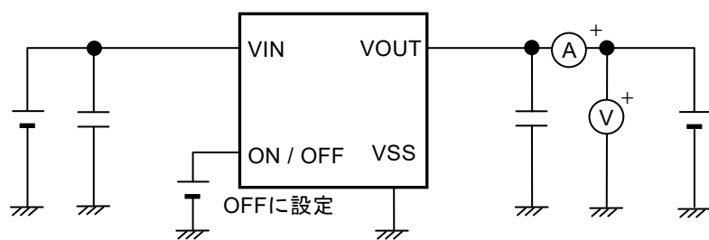
図13 測定回路6
