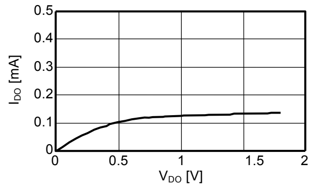
DO端子シンク電流特性 V_{DD} = 1.8\text{ V} , V_M = V_{SS} = 0\text{ V}
