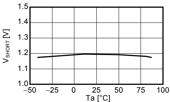
負荷短絡検出電圧-温度特性
