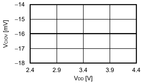
2.11 V_{CIOV} - V_{DD}
