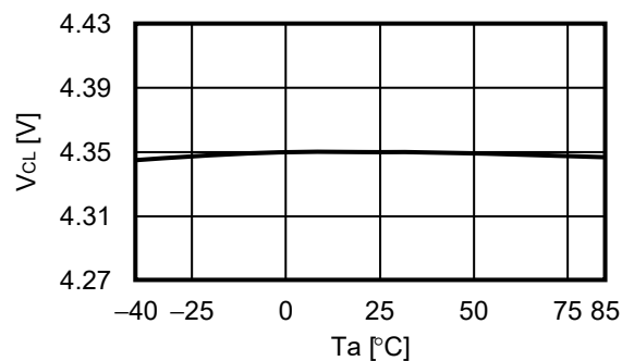
2.2 V_{CL} - T_a
