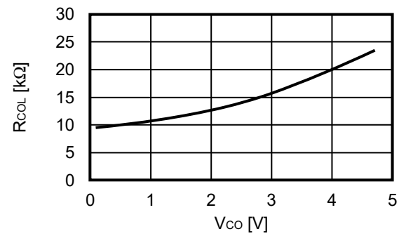
4.2 R_{COL} - V_{CO}
