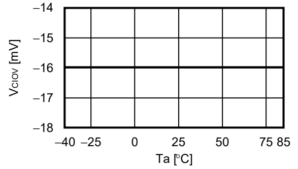
2.12 V_{CIOV} - Ta
