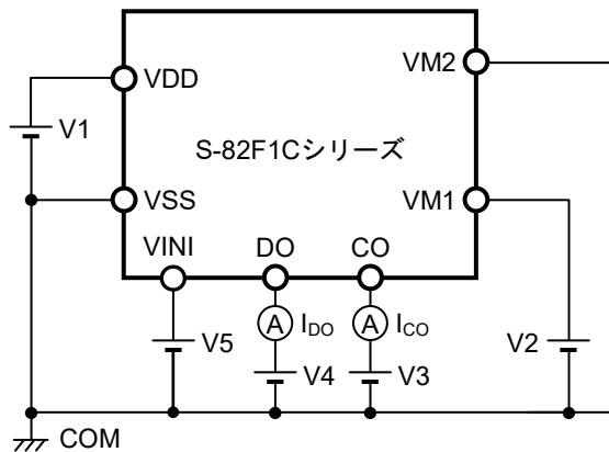
図6 測定回路4
