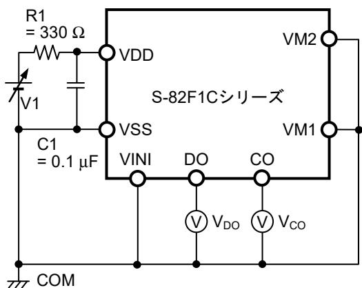
図3 測定回路1
