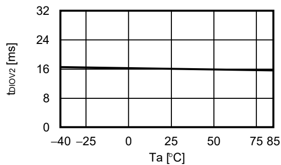
3.6 t_{DIOV2} - T_a
