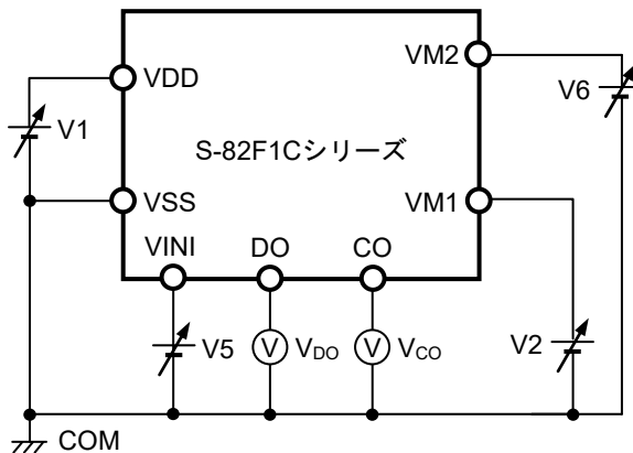
図4 測定回路2
