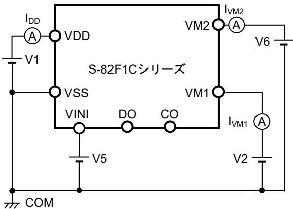
図5 測定回路3
