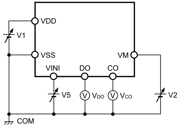
図4 測定回路2
