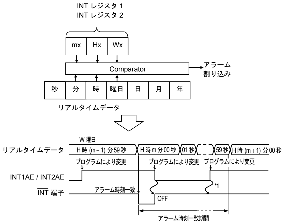
図27 アラーム割り込み出力タイミング
