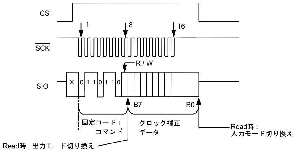
図40 クロック補正レジスタアクセス
