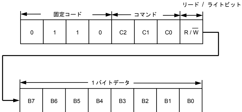
図13 通信データ
