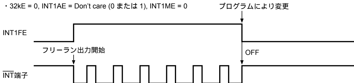
図29 周波数設定出力タイミング
