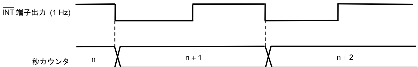
図20 1 Hzのクロック出力と秒カウンタ
