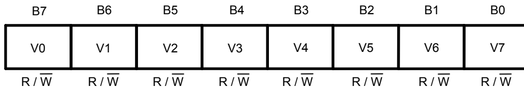
図21 クロック補正レジスタ
