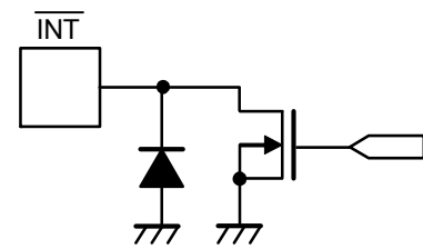
図6 SIO 端子
