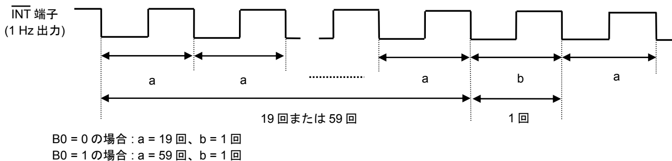
図34 クロック補正確認方法
