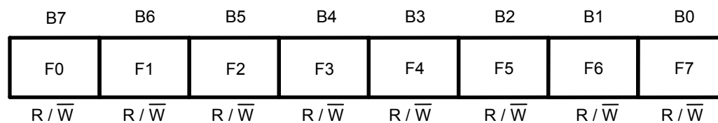
図22 フリーレジスタ
