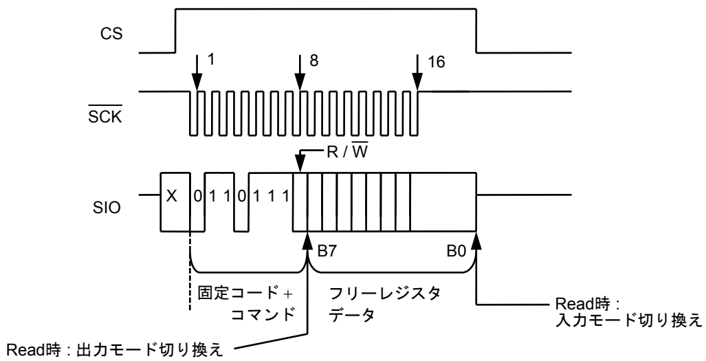
図41 フリーレジスタアクセス
