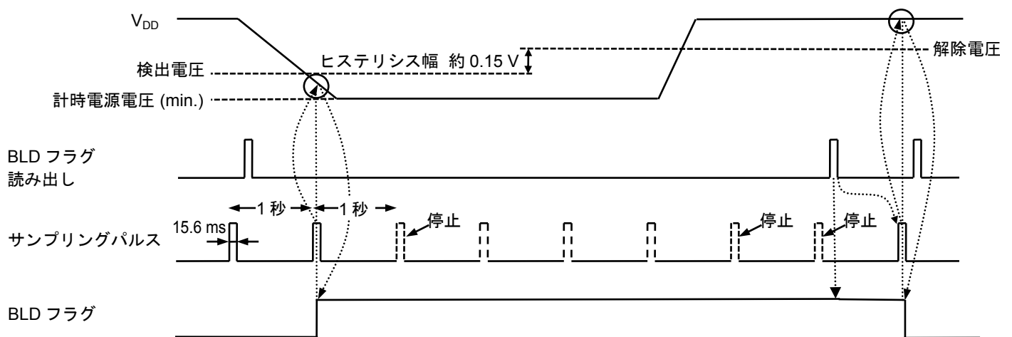
図25 低電源電圧検出回路タイミング
