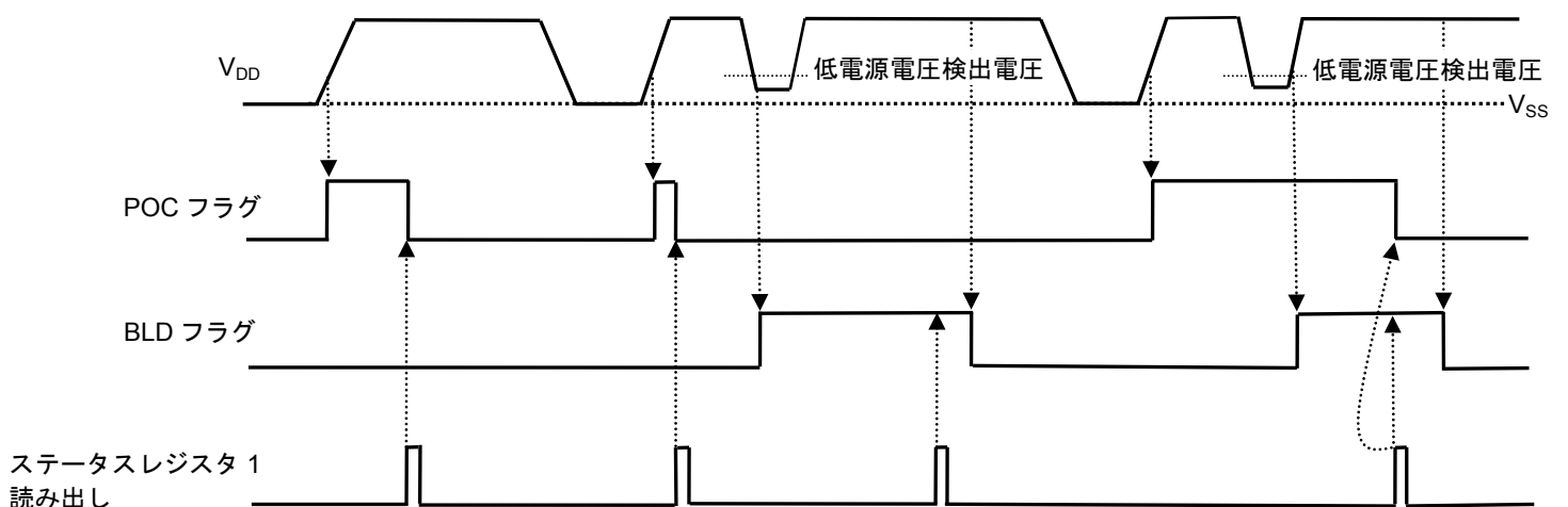
図26 POCフラグとBLDフラグ
