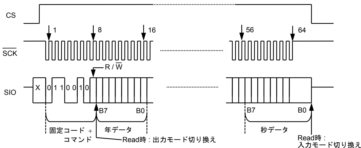
図35 リアルタイムデータ1アクセス
