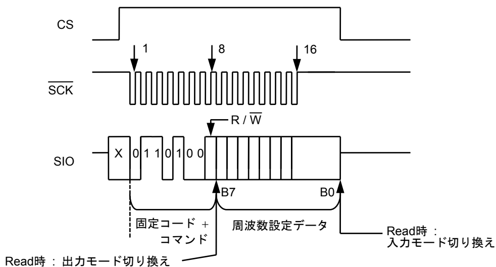
図39 INTレジスタ1(周波数設定データ) アクセス
