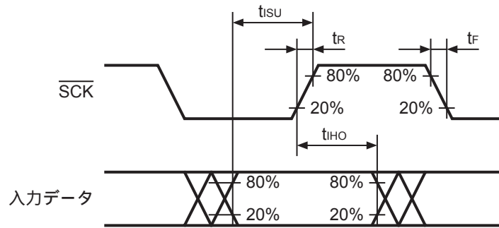
図11 3線式通信のタイミングダイアグラム2
