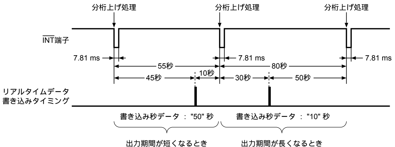
図32 分単位定常割り込み出力2タイミング
