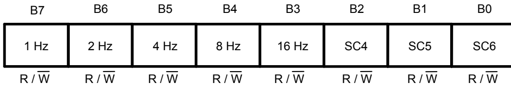
図18 INTレジスタ1 (周波数設定データ)
