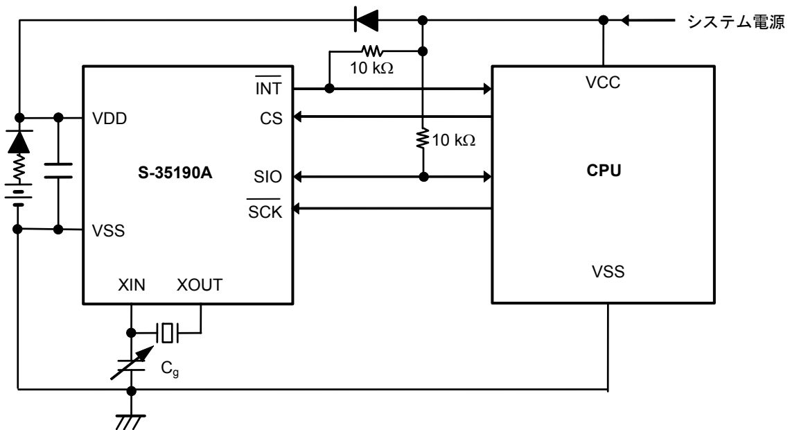
図44 応用回路2
