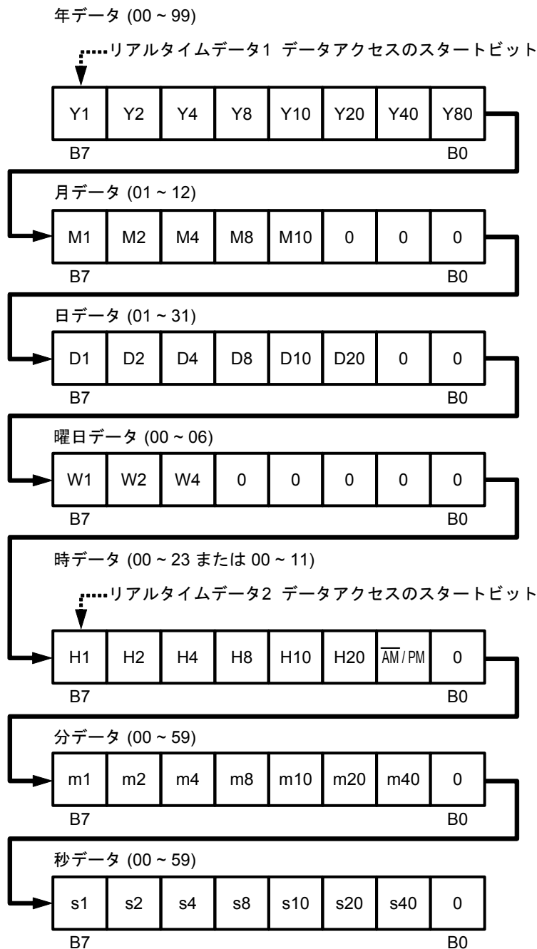
図14 リアルタイムデータレジスタ
