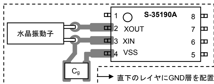
図46 接続図2
