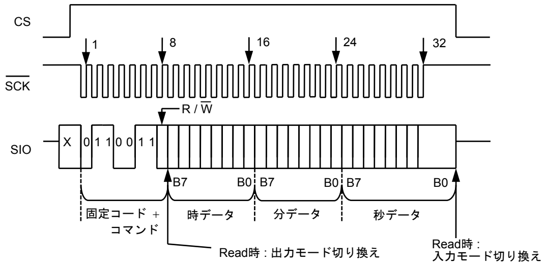
図36 リアルタイムデータ2アクセス
