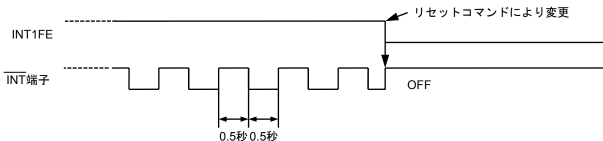
図33 パワーオン検出回路動作時の \overline{\text{INT}} 端子出カタイミング
