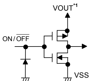
図13 ON/OFF 端子の構造
