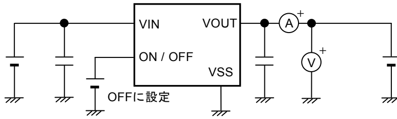
図14 測定回路6
