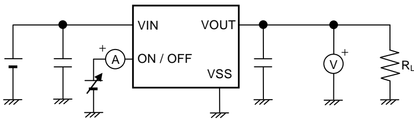
図12 測定回路4
