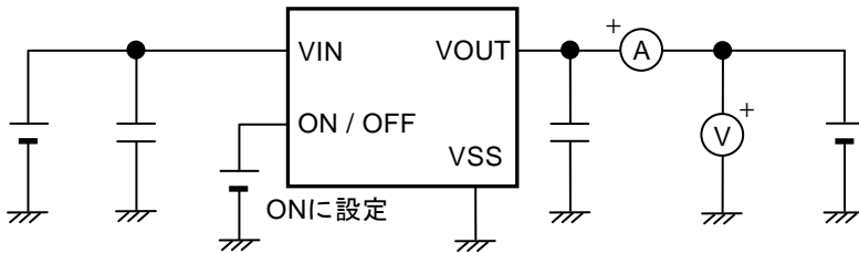
図11 測定回路3
