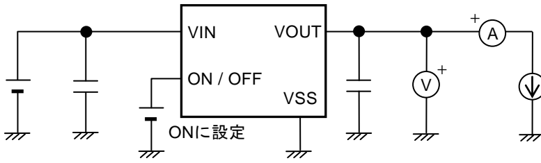
図9 測定回路1
