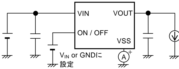
図10 測定回路2
