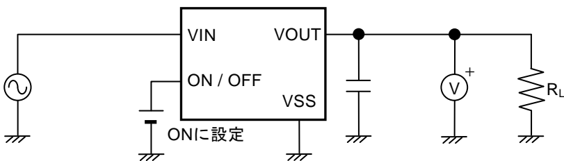
図13 測定回路5
