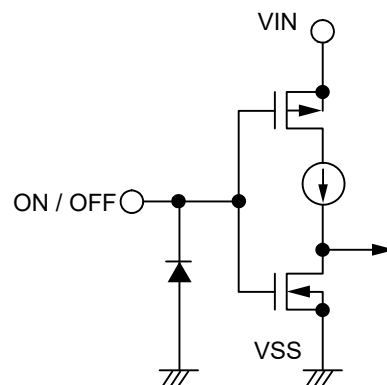
図17 S-1313xxxHシリーズB / Dタイプ
