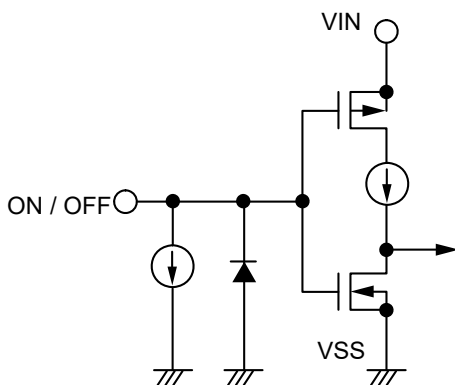
図16 S-1313xxxHシリーズA / Cタイプ
