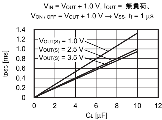
図20 S-1313xxxHシリーズA/Bタイプ (放電シャント機能あり)
