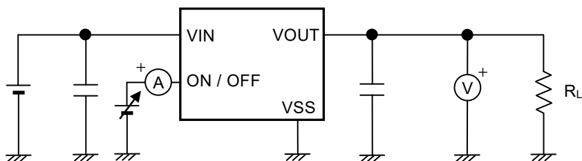
図12 測定回路4
