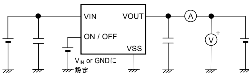
図11 測定回路3
