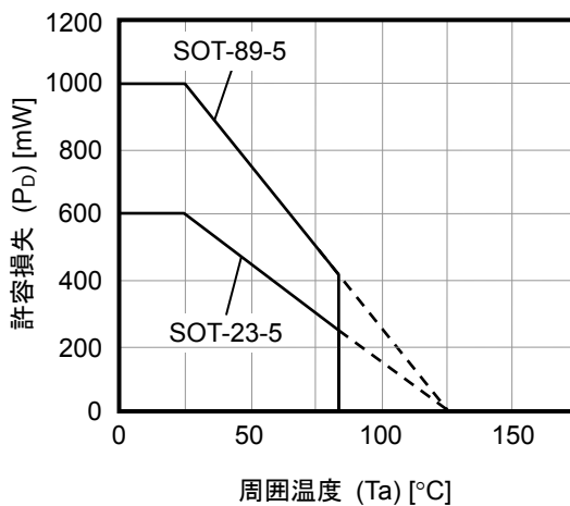
(1) 基板実装時
