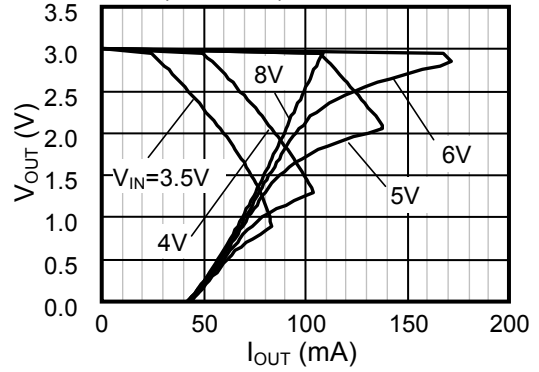
S-812C30B (Ta=25°C) 短絡保護機能あり
