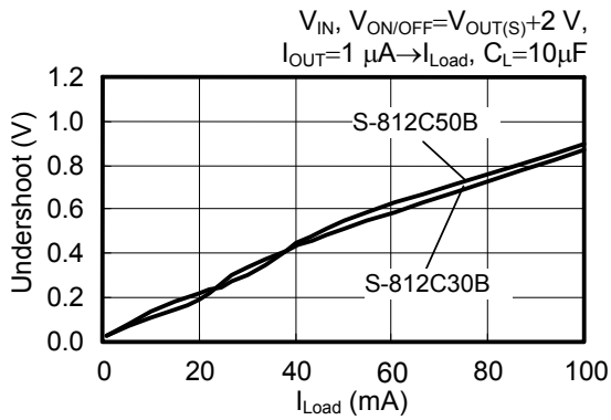
負荷変動アンダーシュートの負荷電流依存性
